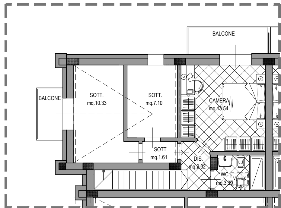
PIANO PRIMO
