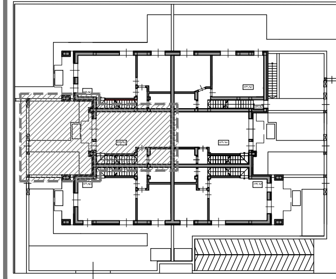
Inquadramento Piano Interrato
